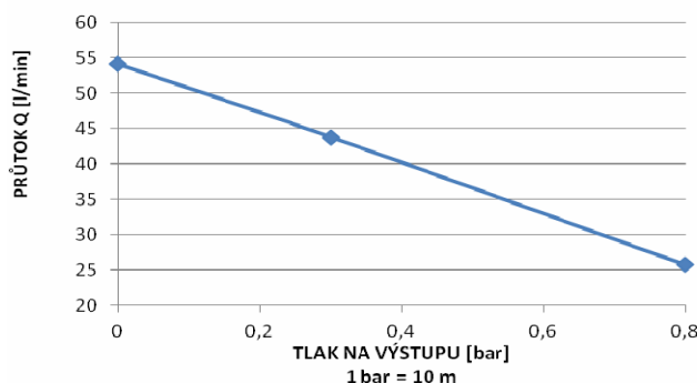
Závislost průtoku a tlaku na výstupu (měřeno při p = 0,4 \text{ MPa} )
