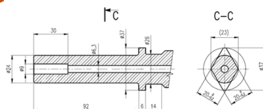
ХВОСТОВИК БУРОВОЙ ШТАНГИ
